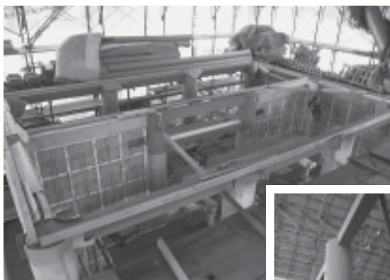
頭貫で繋いだ柱
