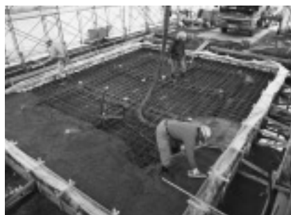
基礎コンクリートの打設
