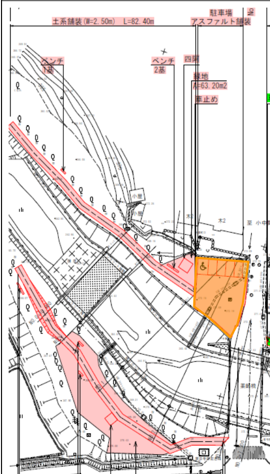
大型バス迂回場所整備平面図
