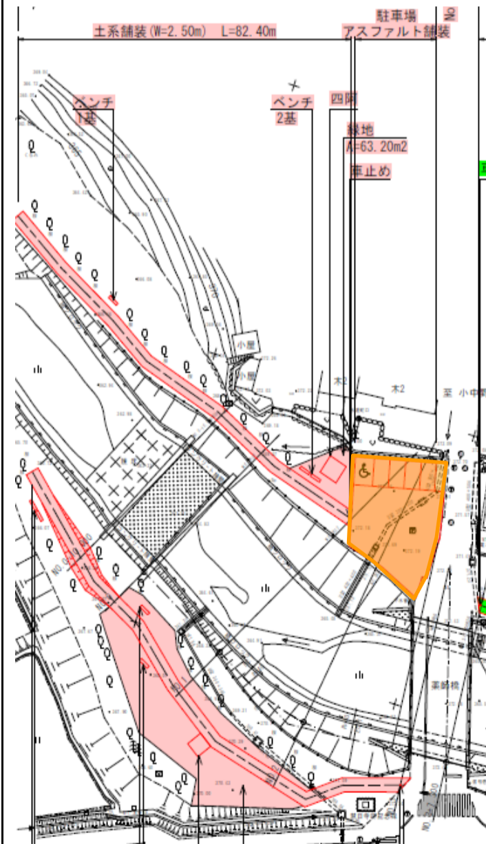
大型バス迂回場所整備平面図
