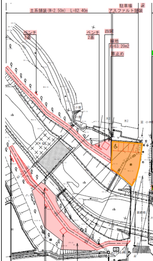
大型バス迂回場所整備平面図
