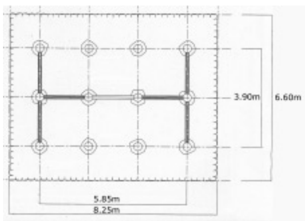
基壇平面図
