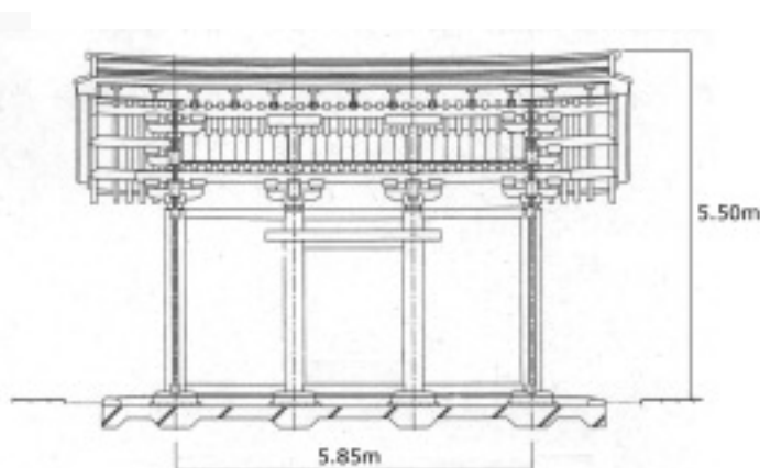
建物立面図
