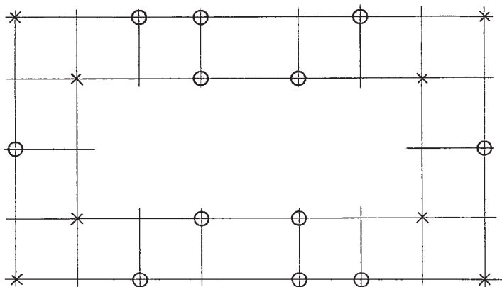
頭貫の継手位置図 (○印、×は組手)
